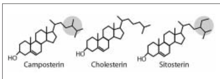
Abbildung: Chemische Struktur von Cholesterin, Camosterin und Sitosterin.
